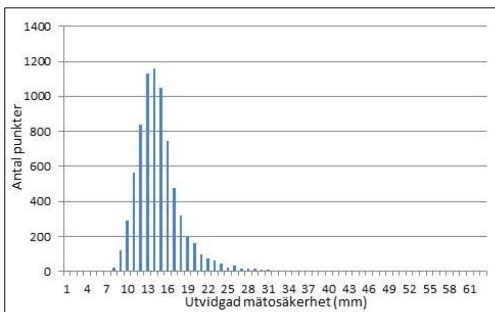
Figur 11: Utvidgad mätosäkerhet i höjd med täckningsgraden 95 %
